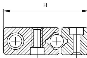
Umlaufkörper
