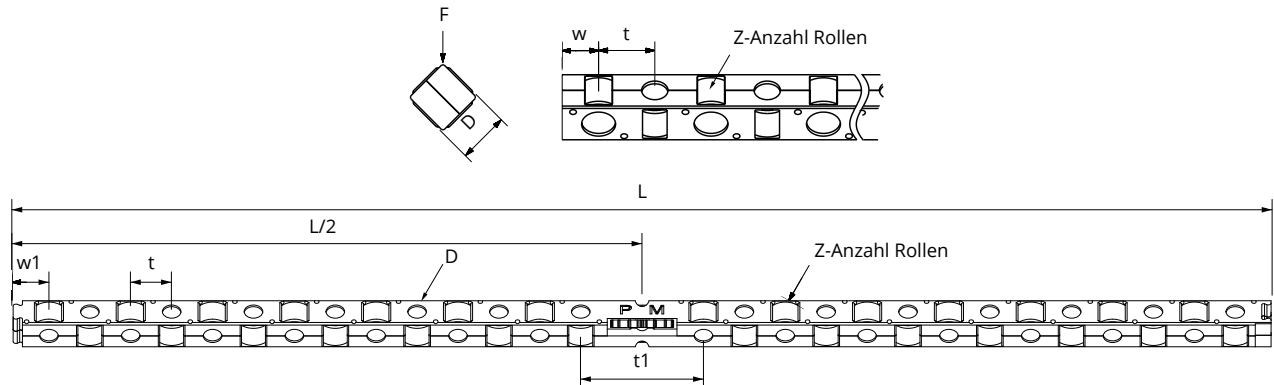
Schnappkäfig
