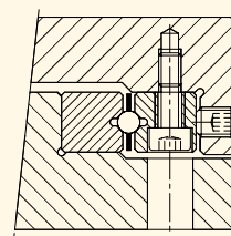
Befestigungsschraube Typ GD
